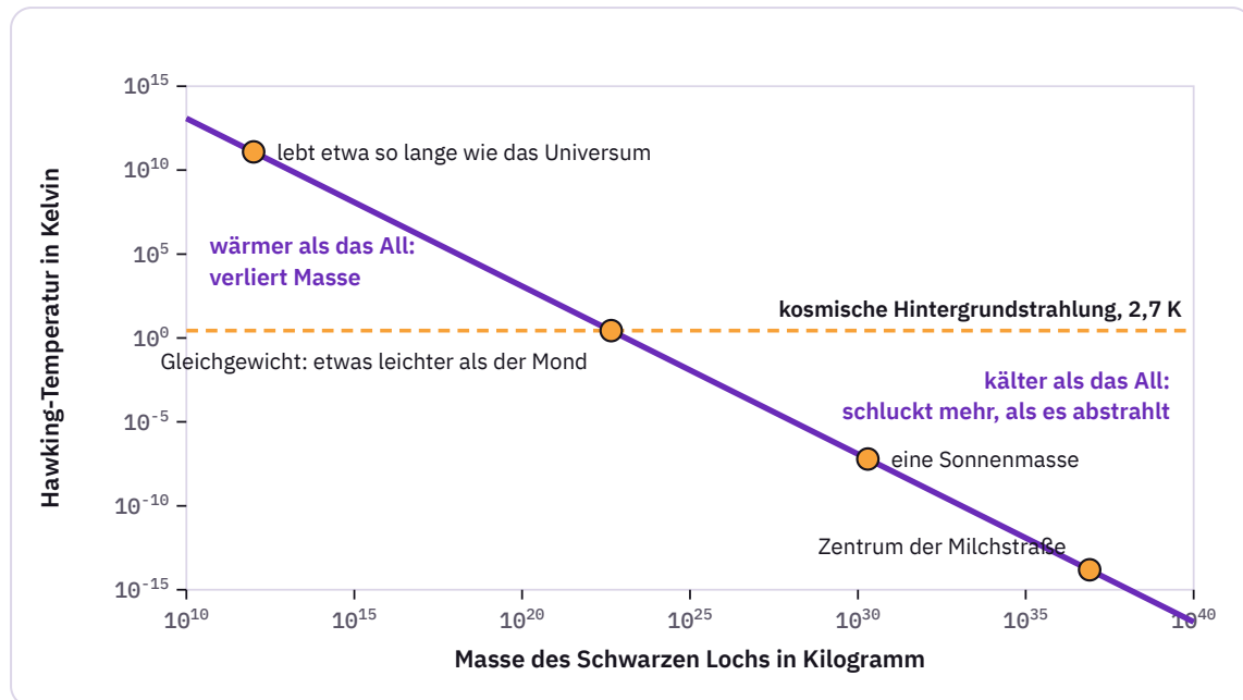
Abb. 1: Je schwerer ein Schwarzes Loch, desto kälter ist es. Eingezeichnet ist die Temperatur der kosmischen Hintergrundstrahlung; das Schwarze Loch im Zentrum der Milchstraße mit rund vier Millionen Sonnenmassen [7] ist um viele Größenordnungen kälter. Eigene Berechnung nach Gleichung (2).
